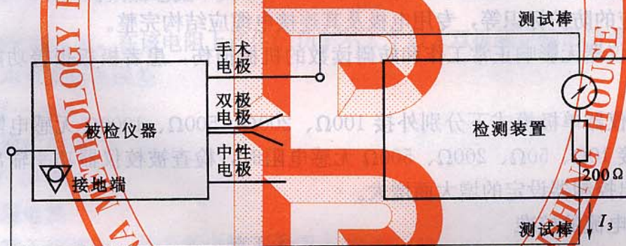
图3 手术电极的高频漏电流
